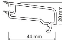
PR7S14B Tek Cam Çıtası Single Glazing Bead
