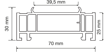
PR7S37 Kasa Yükseltme Profili Frame joint Profile
