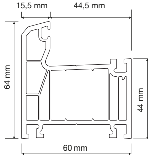
PR6D01 Kasa Profili (5 odacıklı) Frame Profile (5 chambers)
