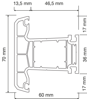
PR6D03 Orta Kayıt 5 Odacıklı Mullion Profile 5 Chamber
