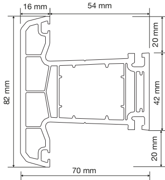
PR7S03 Orta Kayıt Profili Mullion Profile
