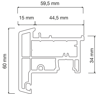
PR6S13 Çift Kanat Adaptörü Overhang(Stump)
