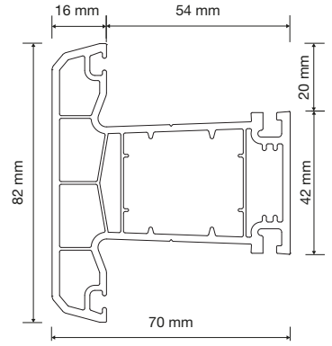
PR7V03B Orta Kayıt Profili Mullion Profile
