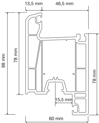
PR6S06 Süper Kapı Profili Super Door Profile
