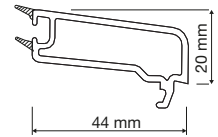
PR7S14B Tek Cam Çıtası Single Glazing Bead
