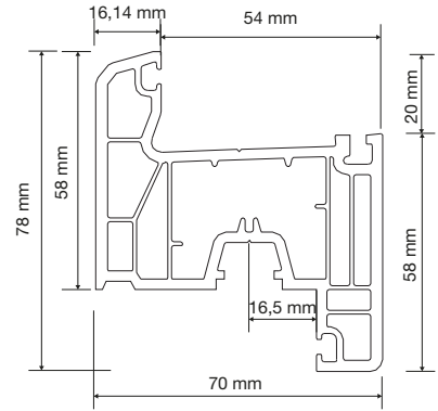
PR7D02 Kanat Profili (5 Odacıklı) Sash Profile (5 Chamber)
