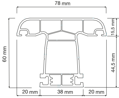
PR6E03 Orta Kayıt Profili Mullion Profile
