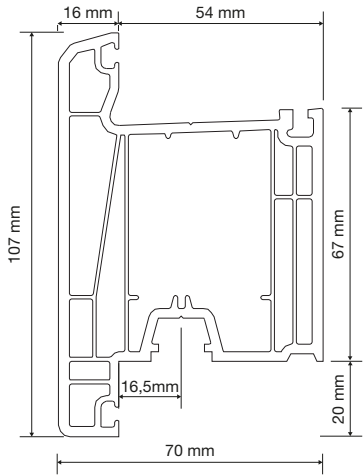
PR7S05B Dışa Açılım Kapı Profili Outside Opening Door Sash Profile
