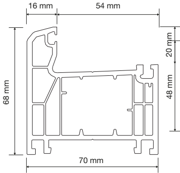
PR7D01 Kasa Profili (5 Odacıklı) Frame Profile (5 Chamber)
