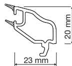
PR7S20 24 mm Dekoratif Çift Cam Çıtası 24 mm Decorative Double Glass Bead
