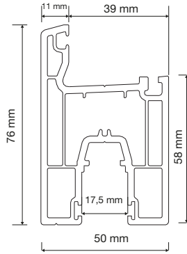
PRSL02 Sürme Kanat Sliding Sash Profile
