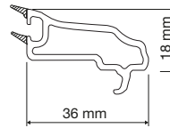
PR6S15B Dekoratif Tek Cam Çıtası Decorative Single Glazing Bead
