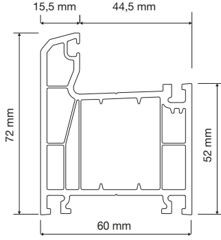
PR6L01 Süper Kasa Profili Super Frame Profile
