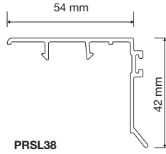
PRSL38 Sürme Kanat Kaplama Sliding Sash Covering
