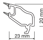
PR7S20 24 mm Dekoratif Çift Cam Çıtası 24 mm Decorative Double Glass Bead
