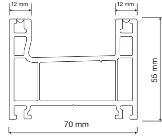
PRSL51 Sürme Çift Raylı Kasa Sliding Double Rail Frame
