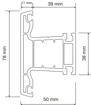
PRSL03 Sürme Orta Kayıt Sliding Mullion Profile
