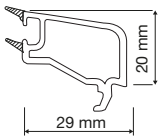
PR7S21B 20 mm Cam Çıtası 20 mm Glazing Bead
