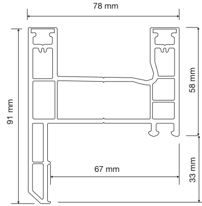
PRSL08 Sürme Pervazlı Kasa Sliding Casing Frame
