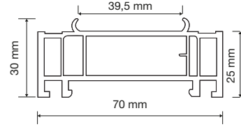
PR7S37 Kasa Yükseltme Profili Frame joint Profile
