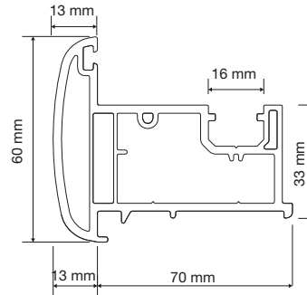
PR7S13B Çift Kanat Adaptör Profili Double Sash Adapter Profile
