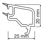
PR7S19 24 mm Çift Cam Çıtası 24 mm Double Glass Bead
