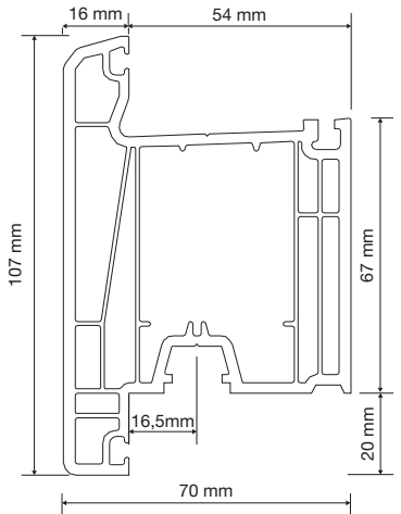
PR7S05B Dış Açılım Kapı Profili Outside Opening Door Sash Profile
