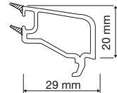
PR7S21B 20 mm Cam Çıtası 20 mm Glazing Bead
