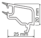
PR7S19 24 mm Çift Cam Çıtası 24 mm Double Glass Bead
