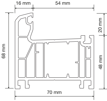
PR7L01 Kasa Profili (6 Odacıklı) Frame Profile (6 Chamber)
