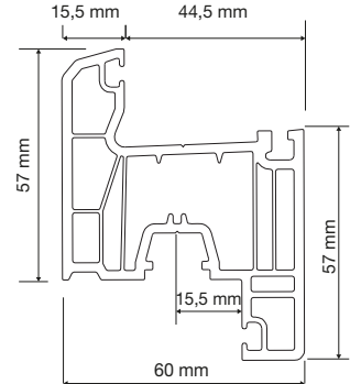
PR6D02 Kanat Profili (5 odacıklı) Sash Profile (5 chambers)
