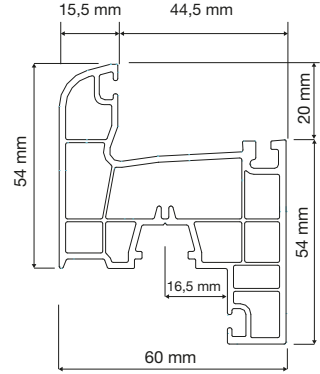
PR6E02 Kanat Profil Sash Profile
