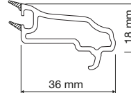
PR6S15B Dekoratif Tek Cam Çitası Decorative Single Glazing Bead
