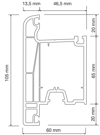
PR6S05 Dış Açılım Kapı Profili Outside Opening Door Sash Profile
