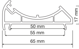
PR6S27 Köşe Dönüş Adaptörü Return Corner Adapter
